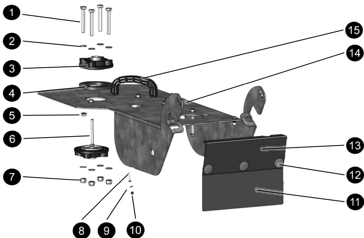
Abbildung 25: Grundrahmen
